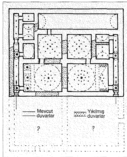
Demirhisar'daki XVI. yüzyıla ait cifte hamamın planı (M. Kiel arşivi)
